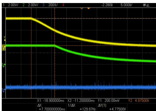
Fig 3. VIN Power OFF(IOUT=0mA)
