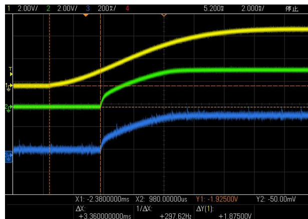
Fig 2. VIN Power ON(IOUT=300mA)
