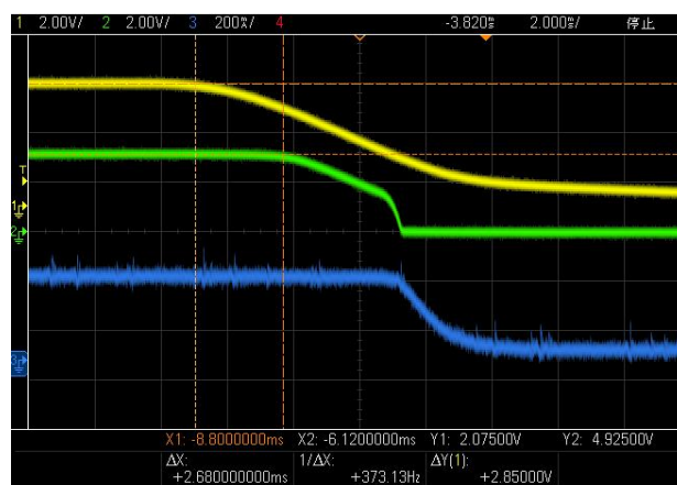
Fig 4. VIN Power OFF(IOUT=300mA)
