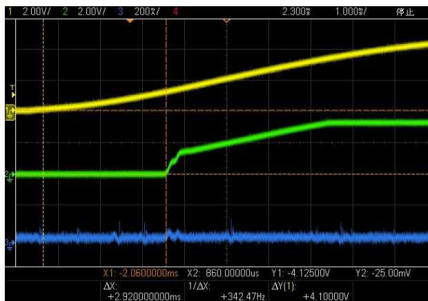
Fig 1. VIN Power ON(IOUT=0mA)
