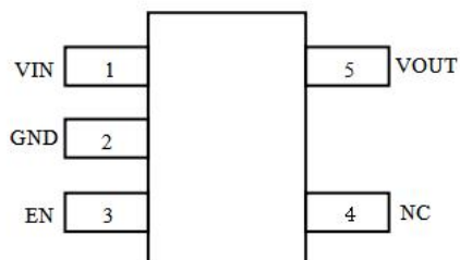
SOT23-5
