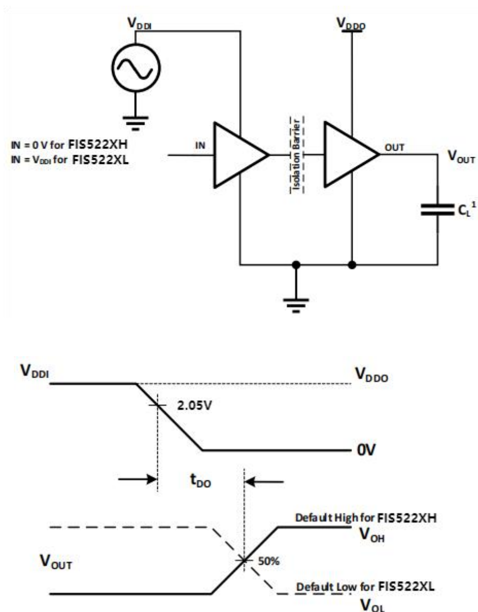
图 3. 默认输出延迟时间测试电路和电压波形
