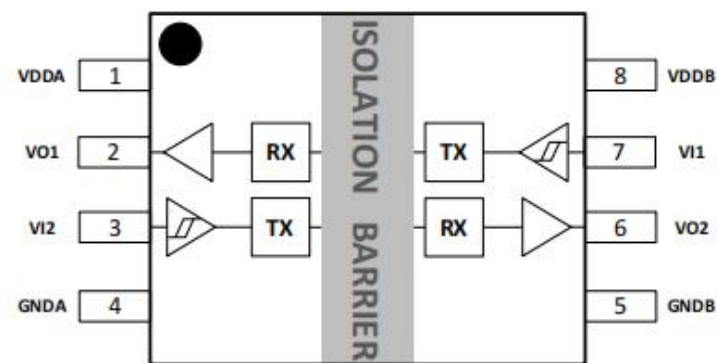
图 1.FIS522X SOW08(宽体)/SOP08(窄体)封装顶部视图
