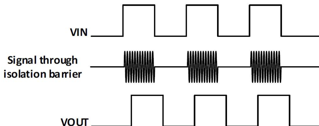
图 6. 00K 开关键控调制方案波形示意图
