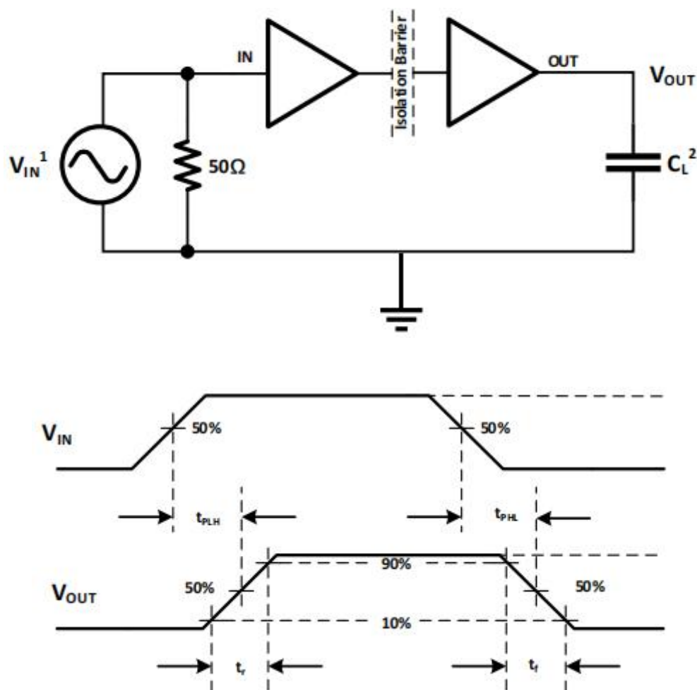
图 2. 时序特性测试电路和电压波形
