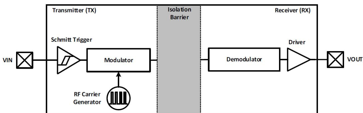
图 5. 单通道功能框图
