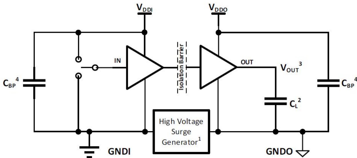
图 4. 共模瞬变抗扰度测试电路
