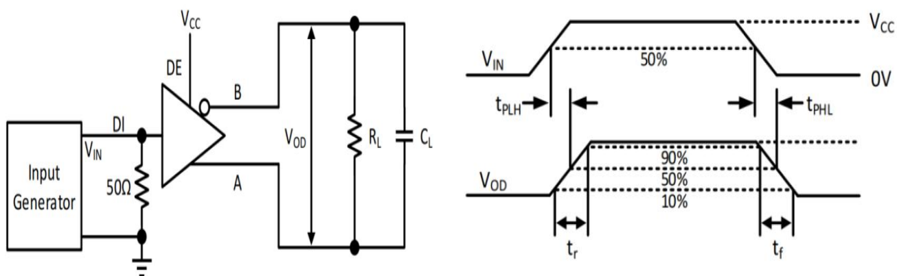
图 21. 测量驱动器差分输出的上升和下降时间以及传播延迟
