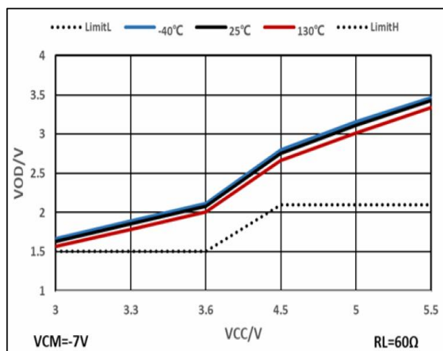
图 2. 共模 -7V 时差分输出电压
