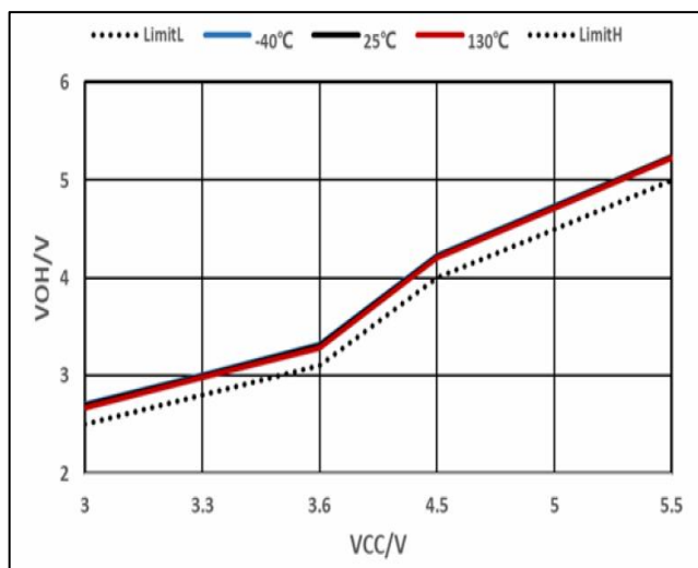
图 7.接收机输出高电平
