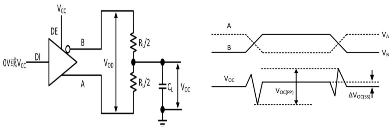
图 19. 使用 RS-485 负载测量驱动器差分 and 共模输出
