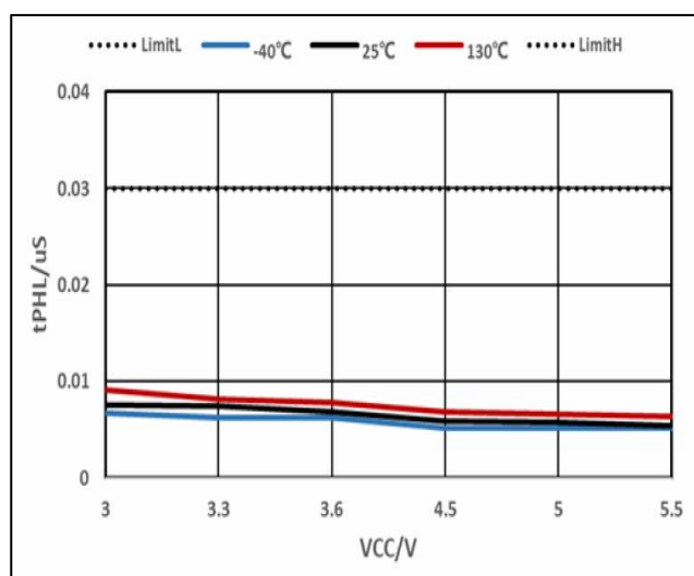
图 10.驱动器输出延迟
