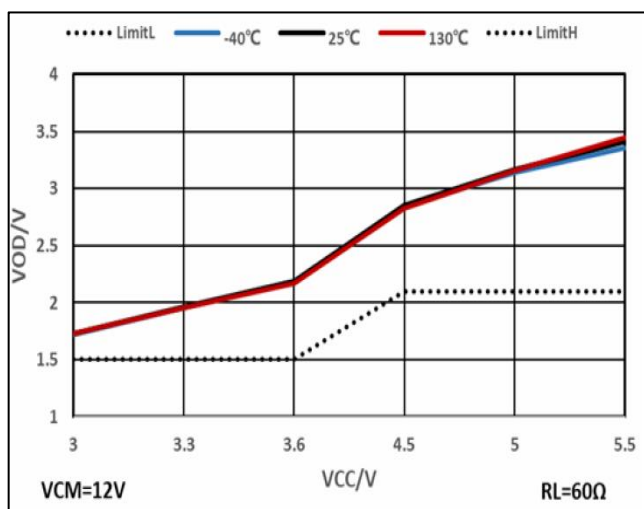
图 1. 共模 12V 时差分输出电压
