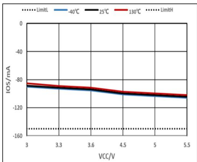
图 17.接收输出短路电流
