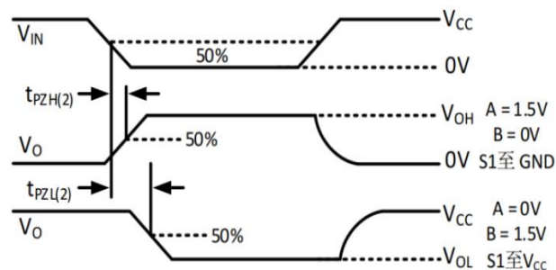
图 25. 在驱动器使能情况下测量接收机使能和关断时间
