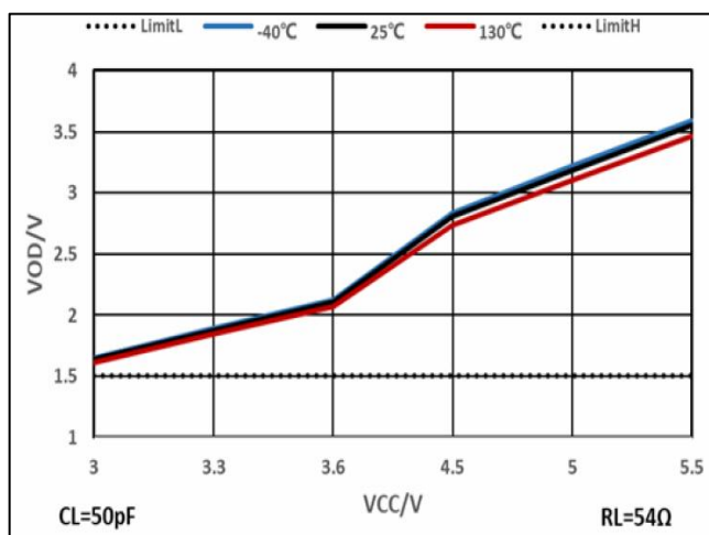
图 3. 54Ω 负载下差分输出电压
