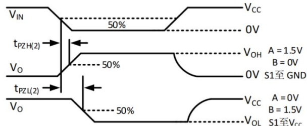
图 26. 在驱动器禁用情况下测量接收机使能时间
