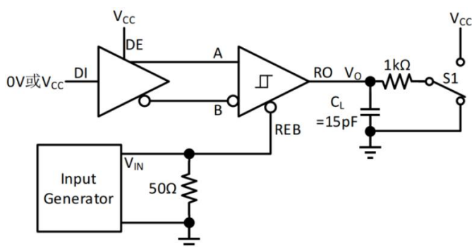
图 25. 在驱动器使能情况下测量接收机使能和关断时间
