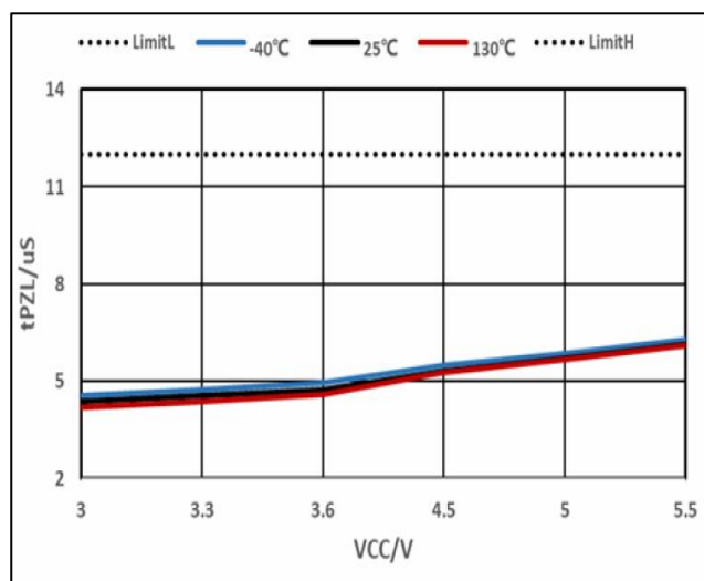
图 12.驱动使能时间
