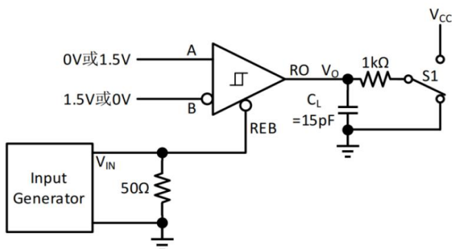
图 26. 在驱动器禁用情况下测量接收机使能时间
