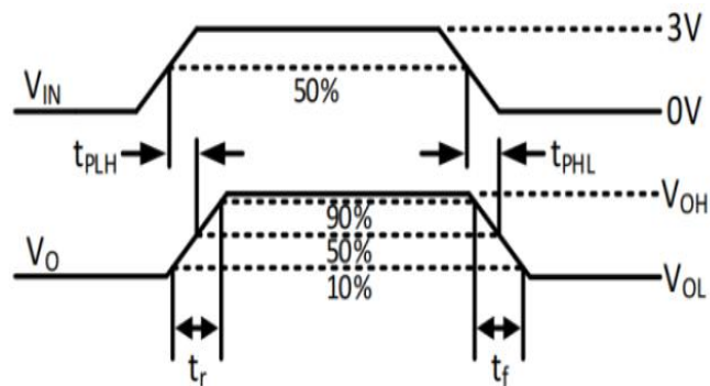
图 24. 测量接收机输出上升和下降时间以及传播延迟
