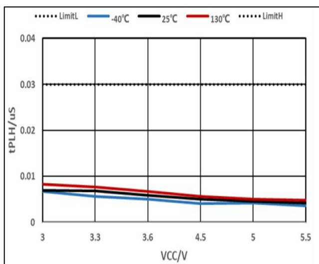
图 9.驱动器输出延迟
