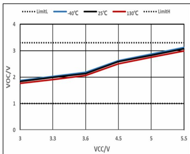
图 6. 100Ω 负载下输出共模电压
