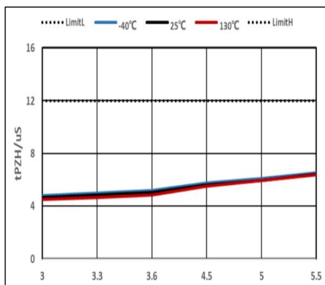
图 16.接收使能时间
