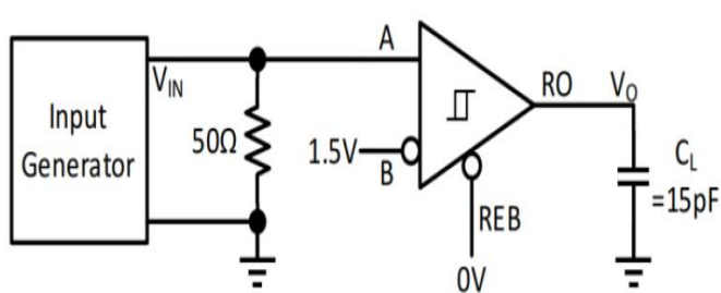
图 24. 测量接收机输出上升和下降时间以及传播延迟
