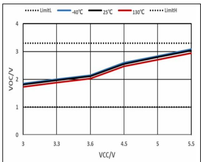
图 5. 54Ω 负载下输出共模电压
