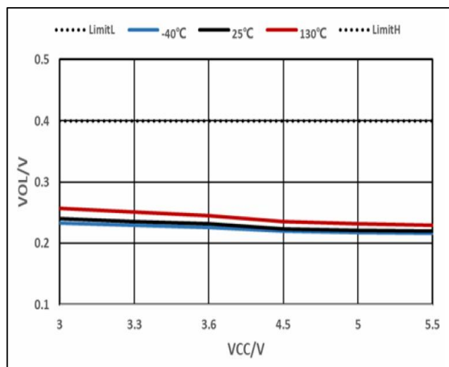
图 8.接收机输出低电平
