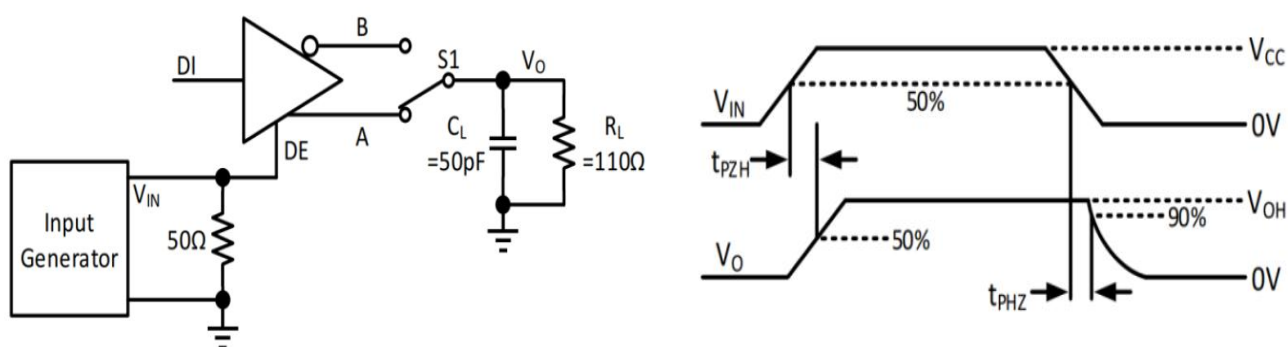
图 22. 在有效高电平输出和下拉负载情况下测量驱动器使能和关断时间
