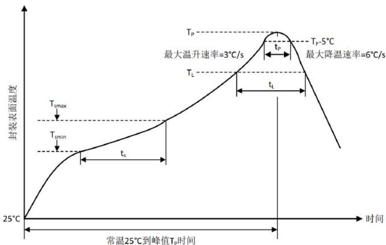
图 28. 焊接温度曲线
