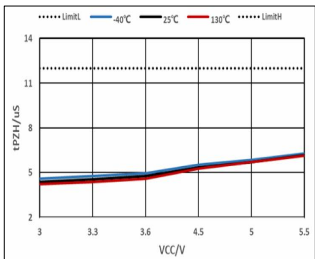
图 11.驱动使能时间
