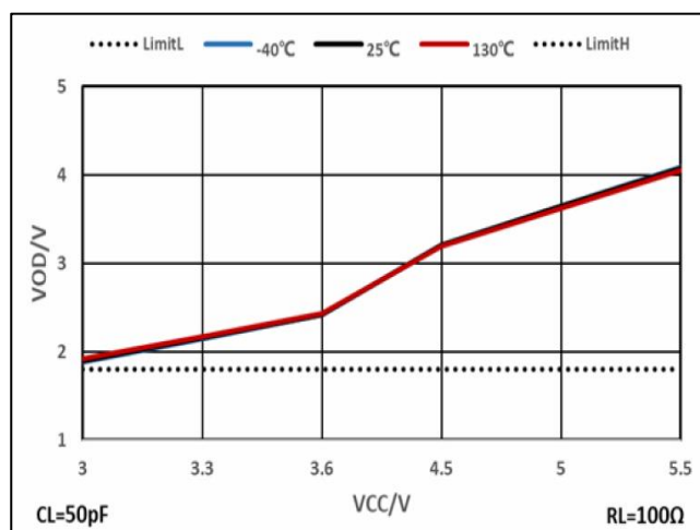
图 4. 100Ω 负载下差分输出电压
