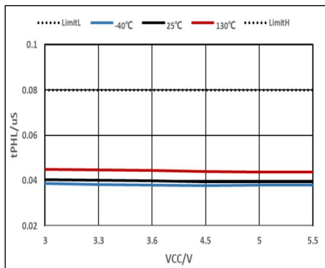
图 14.接收传输延时
