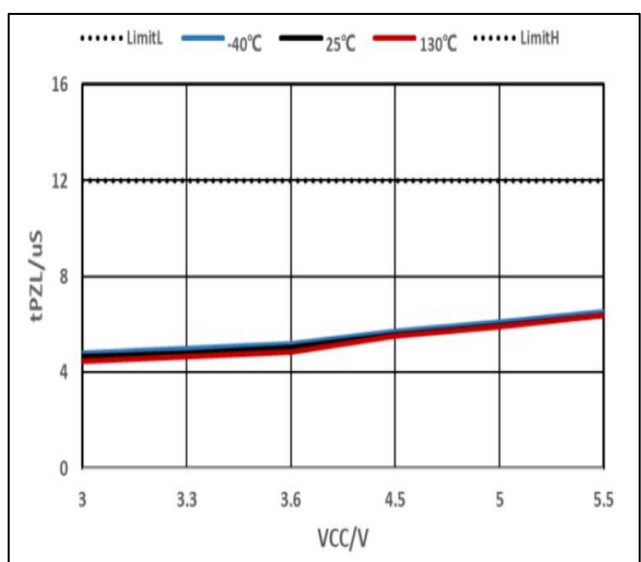
图 15.接收使能时间
