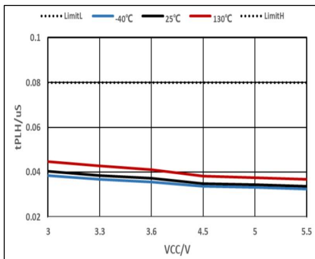
图 13.接收传输延时
