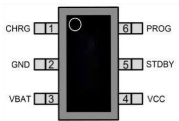
SOT23-6L
