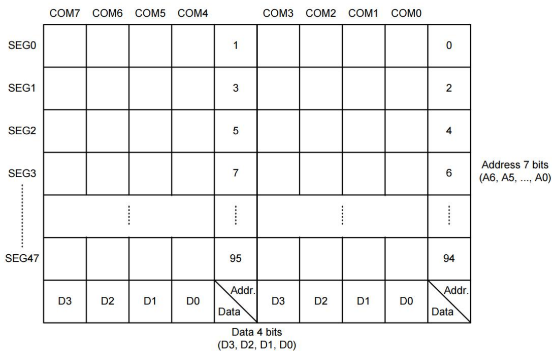
RAM 映射
